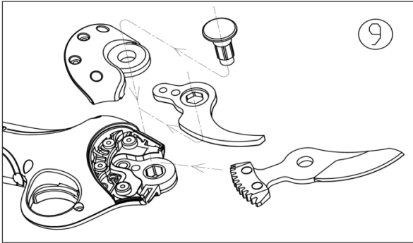
9. Messersatz montieren, Deckel aufsetzen und Zentrierbolzen einsetzen.
