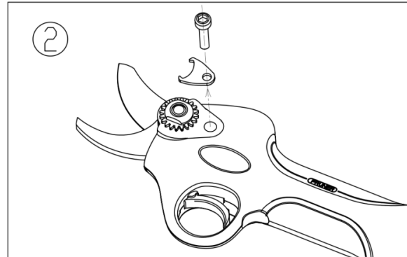
2. Entfernen Sie die Schraube der Einstellklammer und die Einstellklammer
