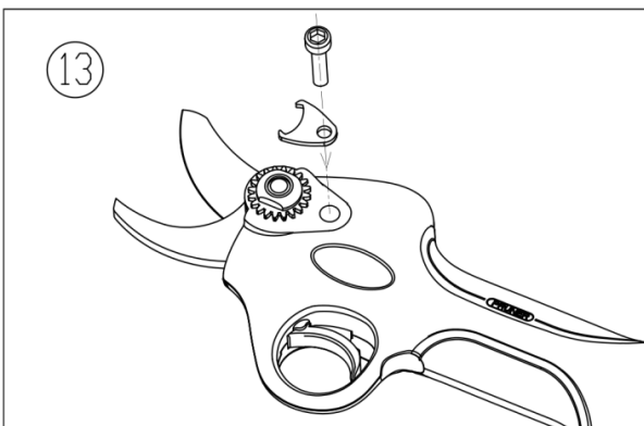
13. Sichern Sie die Überwurfmutter mit Clip und Steckbolzen.
