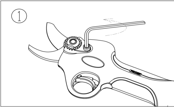
1. Lösen Sie die Einstellschraube mit einem Inbusschlüssel.
