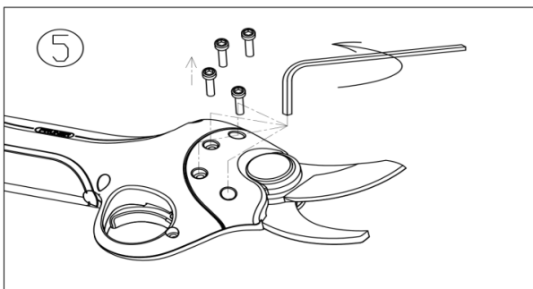
5. Dévisser les 4 vis du couvercle à l'aide d'une clé Allen.
