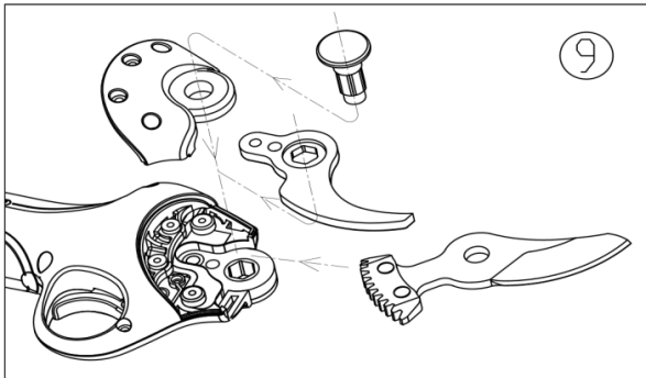
9. Assemblare il set di lame, posizionare il coperchio e inserire il bullone centrale.
