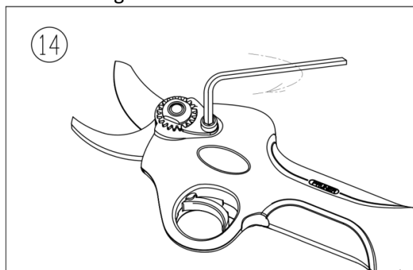
14. Stringere la vite di regolazione.
