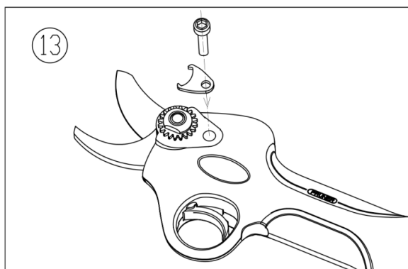
13. Fissare il dado dell'ingranaggio con la clip e inserire il vite della clip dell'ingranaggio.
