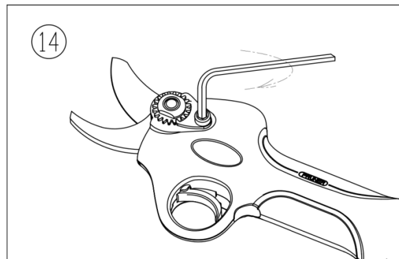
14. Ziehen Sie die Klemmschraube der Getriebemutter an, die die Getriebemutter der Zentrierbolzen befestigt.
