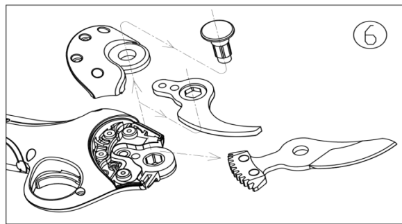
6. Retirer le couvercle et démonter le jeu de lames.
