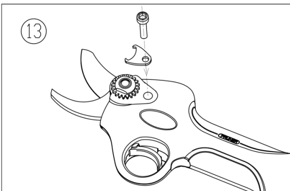
13. Fixer l'écrou du réducteur à l'aide d'un clip et d'un boulon d'insertion.
