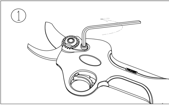
1. Desserrer le boulon du clip de réglage à l'aide d'une clé Allen.
