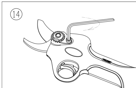
14. Serrer le clip de serrage de l'écrou en sécurisant l'écrou de l'engrenage central.
