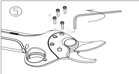
5. Desatornille los 4 tornillos de la tapa con una llave Allen.
