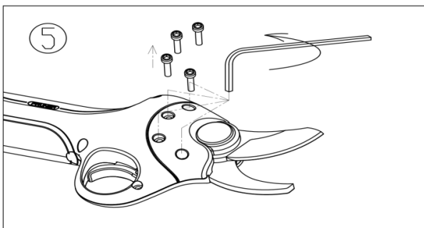
5. 4 Deckelschrauben mit Inbusschlüssel lösen.
