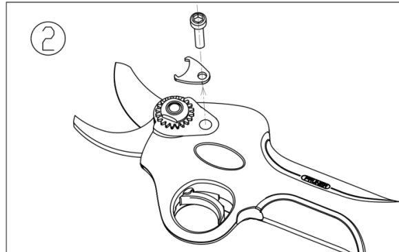
2. Quite el perno del clip de ajuste y el clip de ajuste.
