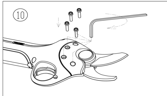
10. Serrer les 4 vis du couvercle à l'aide d'une clé Allen.
