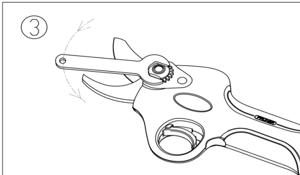
3. Lösen Sie die Überwurfmutter mit einem Schraubenschlüssel.
