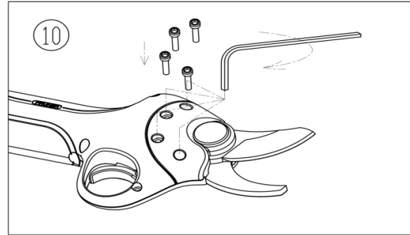
10. 4 Deckelschrauben mit Inbusschlüssel anziehen.
