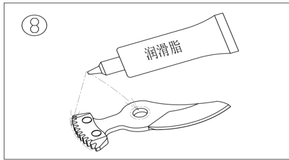
8. Appliquer de la graisse sur les dents de l'engrenage et le trou du boulon central.
