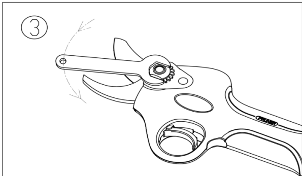
3. Desserrer l'écrou du réducteur à l'aide d'une clé.
