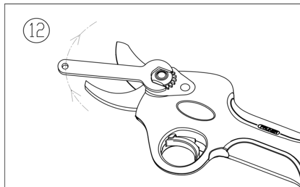
12. Serrer l'écrou à l'aide d'une clé à molette.
