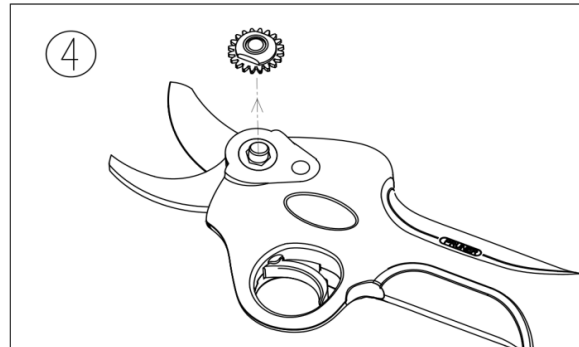
4. Retirer l'écrou de réglage.
