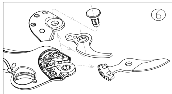
6. Entfernen Sie die Abdeckung und demontieren Sie den Messersatz.
