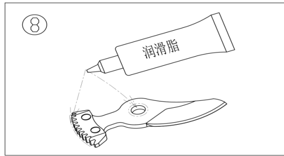
8. Tragen Sie Fett auf die Verzahnung und das Loch für die Zentrierbolzen auf.
