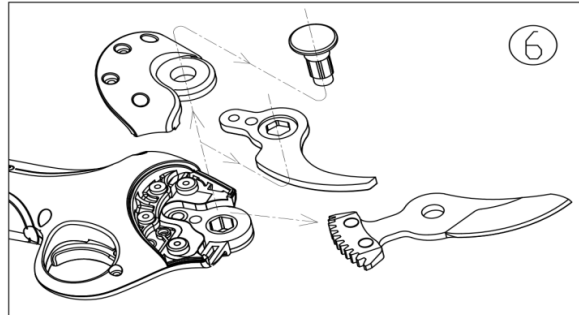
6. Quite la tapa y desmonte el juego de la hoja.
