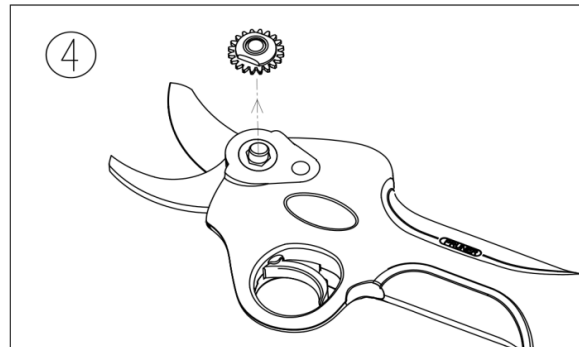
4. Quite la tuerca del engranaje de ajuste.
