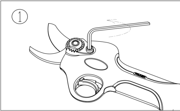
1. Afloje el perno del clip de ajuste con una llave Allen
