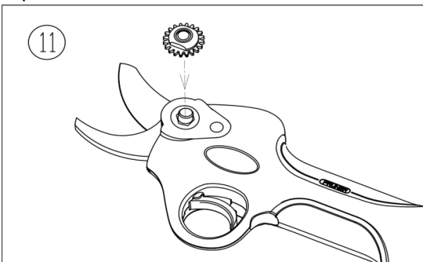
11. Posizionare il dado dell'ingranaggio sul bullone centrale.
