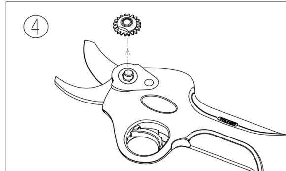
4. Einstelltriebemutter entfernen.
