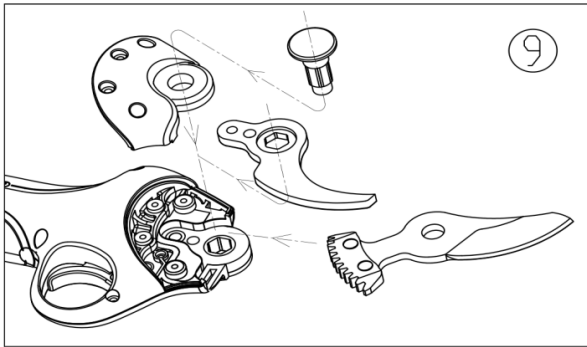
9. Assembler le jeu de lames, placer le couvercle et insérer le boulon central.
