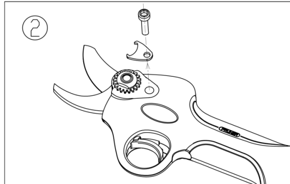
2. Retirer le boulon du clip de réglage et le clip de réglage.
